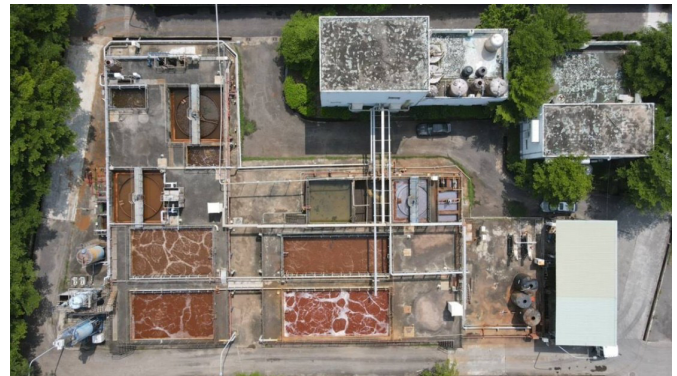
安定滲出水處理廠
