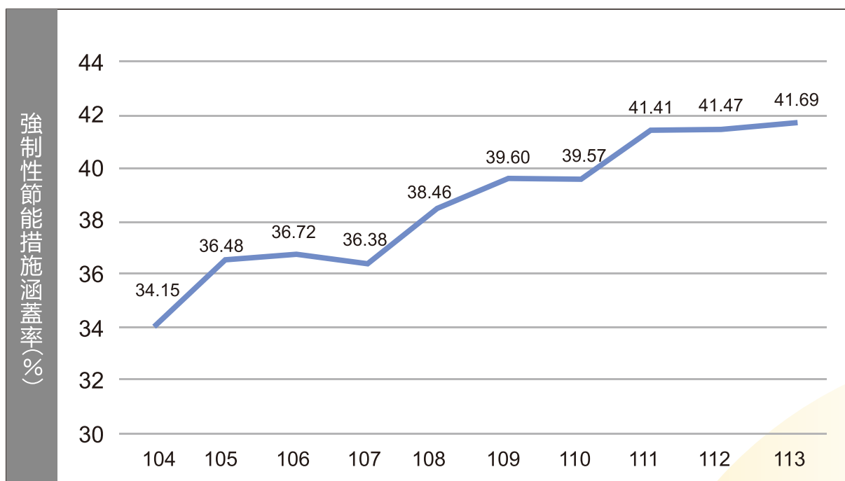
▲ 圖2-14 我國各年度強制性節能措施涵蓋率
