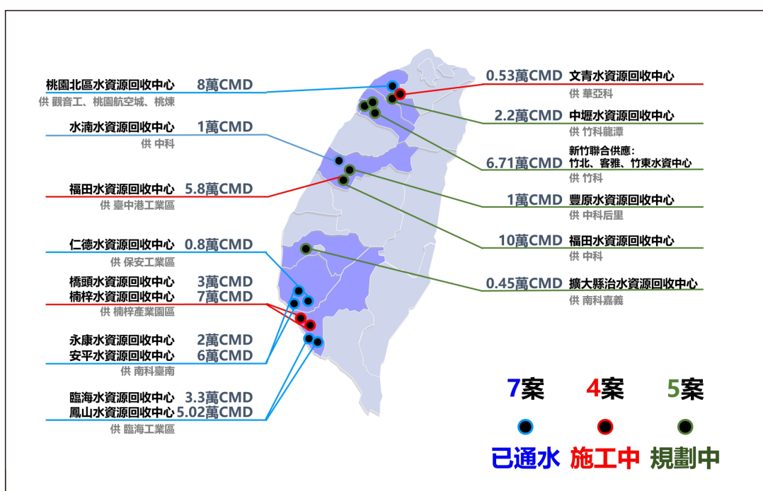
▲ 圖2-10 再生水建設成果圖
